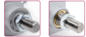
K5 Mil Keçesi Teknopolimer Sıyrıcı (POM+PU)
